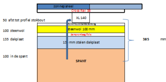
Figuur 1: schematische weergave van de dakconstructie
